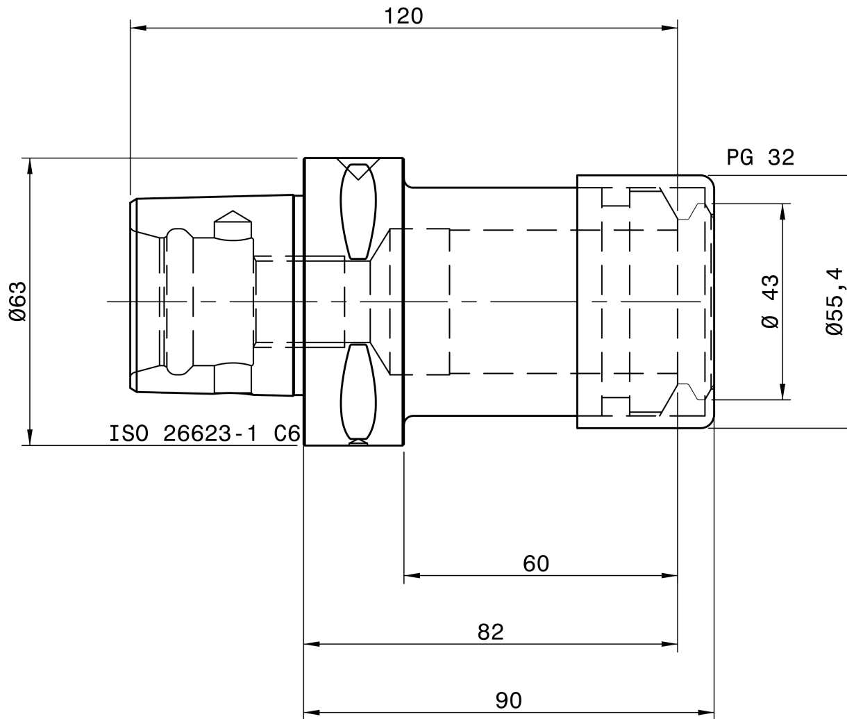
REGO-FIX SG 5806.73240
