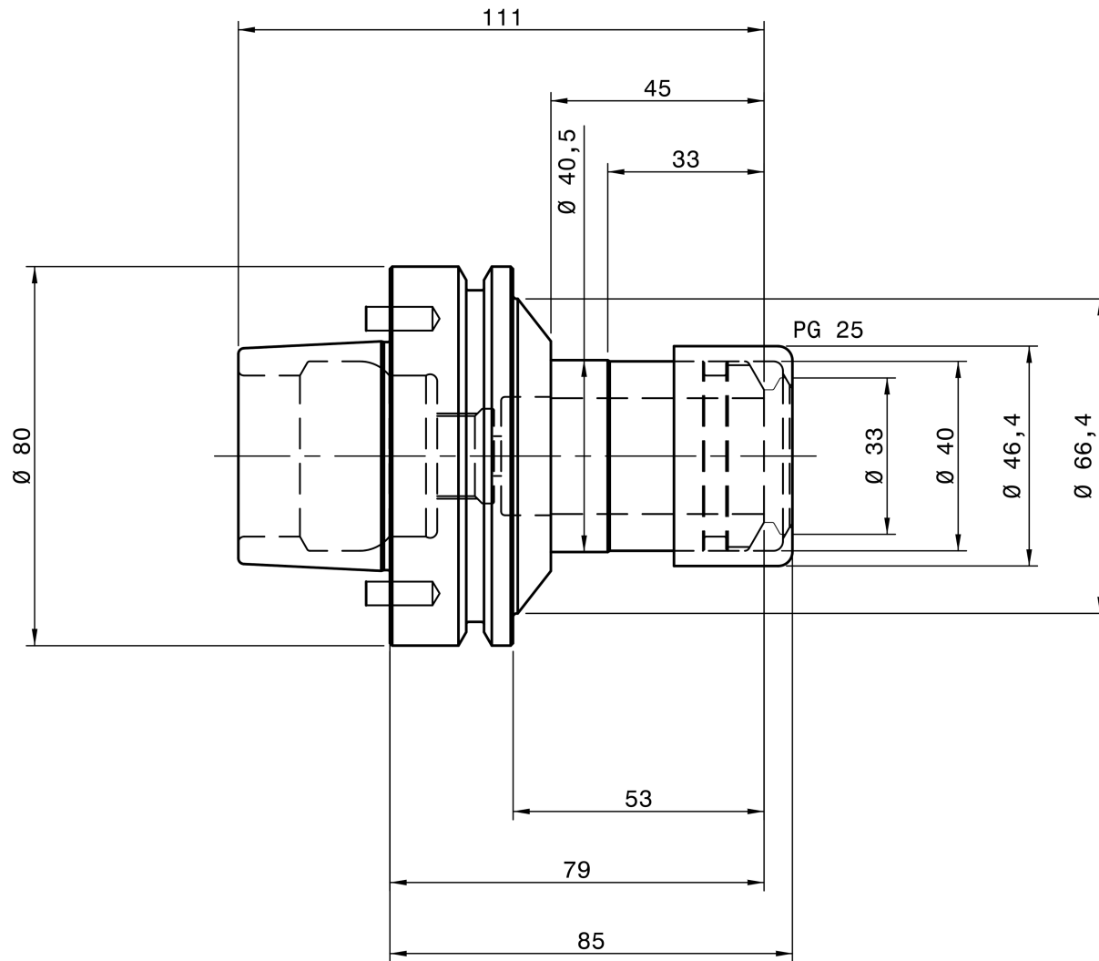
REGO-FIX 8070.80250
