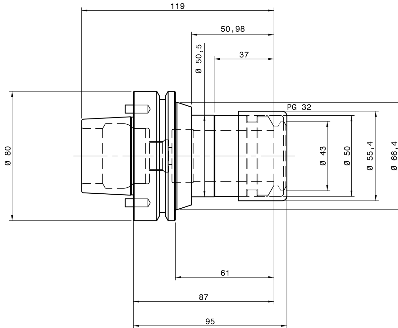
REGO-FIX 8070.80320
